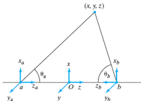
图 13.10: 同核双原子分子的坐标系统。
